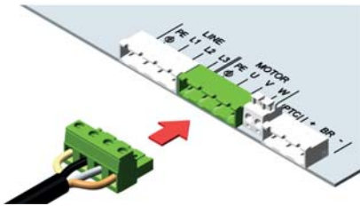
Электрическое соединение
