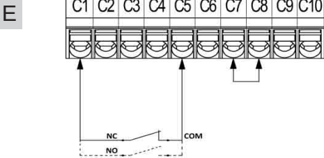
Conexión eléctrica
