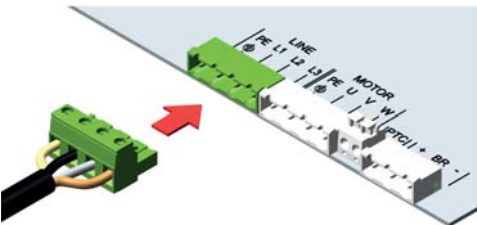
Collegamento elettrico
