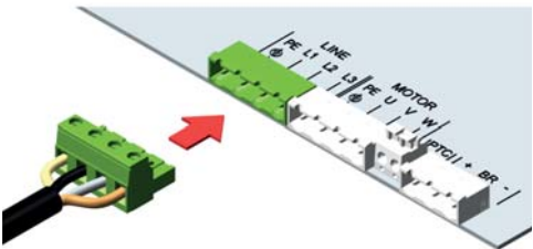
Conexión eléctrica
