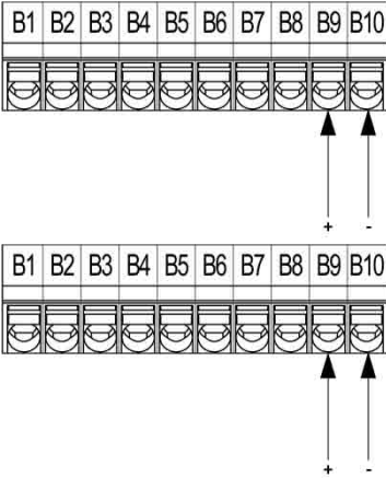
Conexión eléctrica
