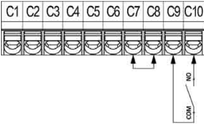
Conexión eléctrica
