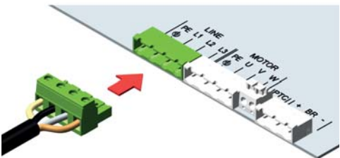
Электрическое соединение
