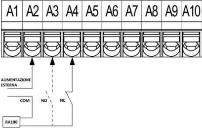
Conexión eléctrica alarma proporcionada
